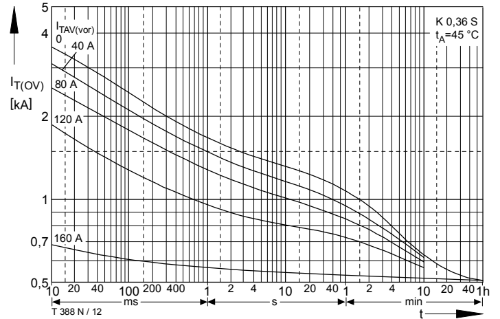
Bild / Fig. 12 Überstrom / Overload on-state current I_{T(OV)} = f(t) Luftselbstkühlung / Natural air-cooling t_A = 45 °C Kühlkörper / Heatsink: K0.36S Parameter: Vorlaststrom / Pre-load current I_{TAV(vor)}
