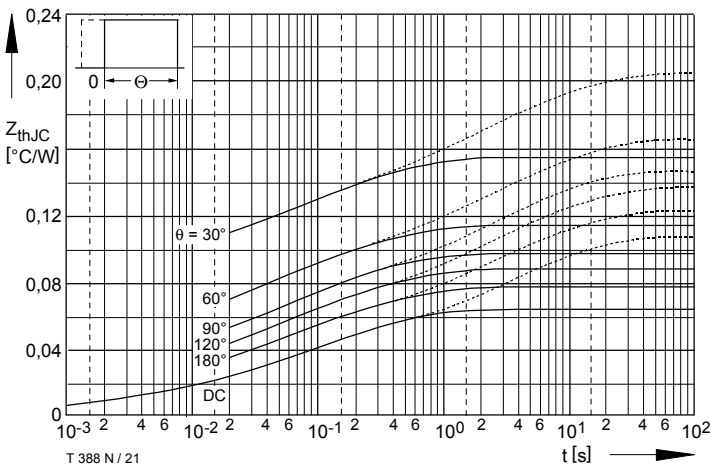
Bild / Fig. 21 Transienter innerer Wärmewiderstand / Transient thermal impedance Z_{thJC} = f(t) - - - - - Anodenseitige Kühlung / Anode-sided cooling ———— Beidseitige Kühlung / Two-sided cooling Parameter: Stromflußwinkel / current conduction angle \theta
