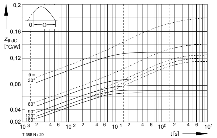
Bild / Fig. 20 Transienter innerer Wärmewiderstand / Transient thermal impedance Z_{thJC} = f(t) - - - - - Anodenseitige Kühlung / Anode-sided cooling ———— Beidseitige Kühlung / Two-sided cooling Parameter: Stromflußwinkel / current conduction angle \theta
