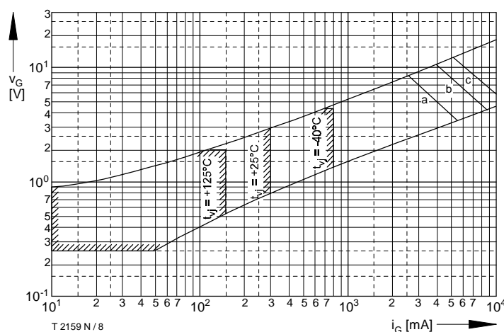
Bild / Fig. 8 Steuercharakteristik mit Zündbereichen / Gate characteristic with triggering areas v_G = f(i_G) , V_D = 6 \text{ V} Parameter: Steuerimpulsdauer / Puls duration t_p [ms] a b c Höchstzulässige Spitzensteuerleistung / Maximum allowable peak gate power [W] 20 40 60
