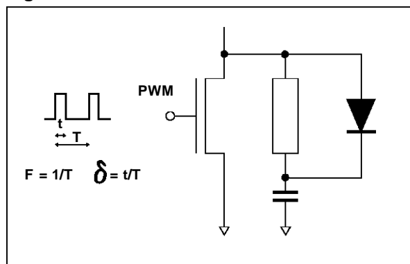
Fig. 2 : SNUBBER DIODE.
