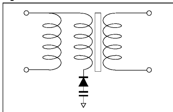
Fig. 4 : DEMAGNETIZING DIODE.
