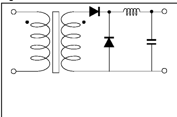
Fig. 5 : RECTIFIER DIODE.
