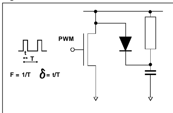
Fig. 3 : CLAMPING DIODE.
