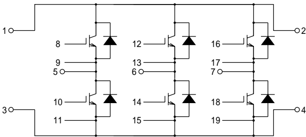
回路図 CIRCUIT
