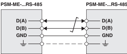
RS-485 interface
