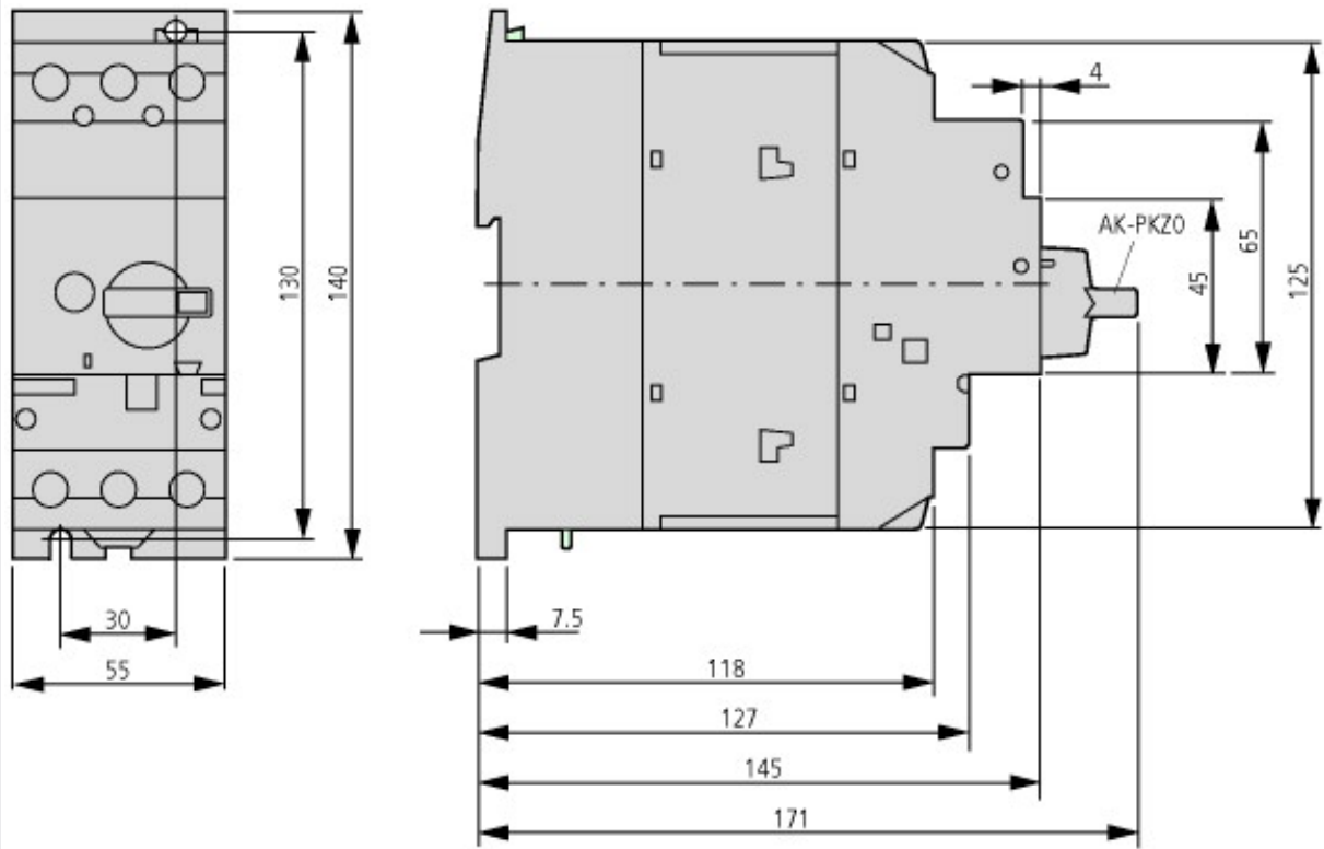
PKZM4-... +AK-PKZ0
