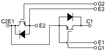
回路図 CIRCUIT
