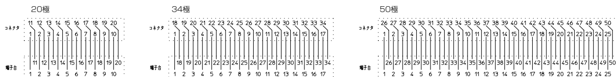
結線図
