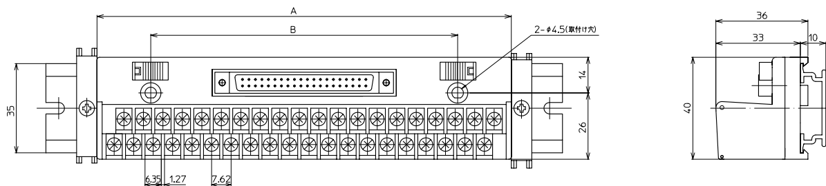
実装コネクタ
