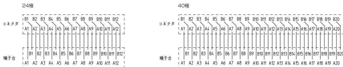
結線図 (TOP VIEW)
