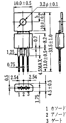
T-4 (13-10A1A)
