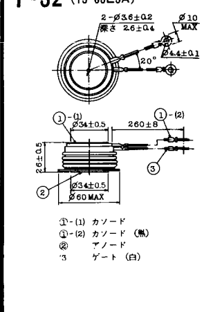
T-32 (13-60E3A)
