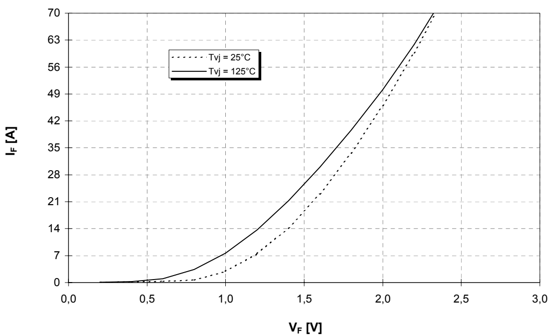
Durchlaßkennlinie der Inversdiode (typisch) ( V_F )
