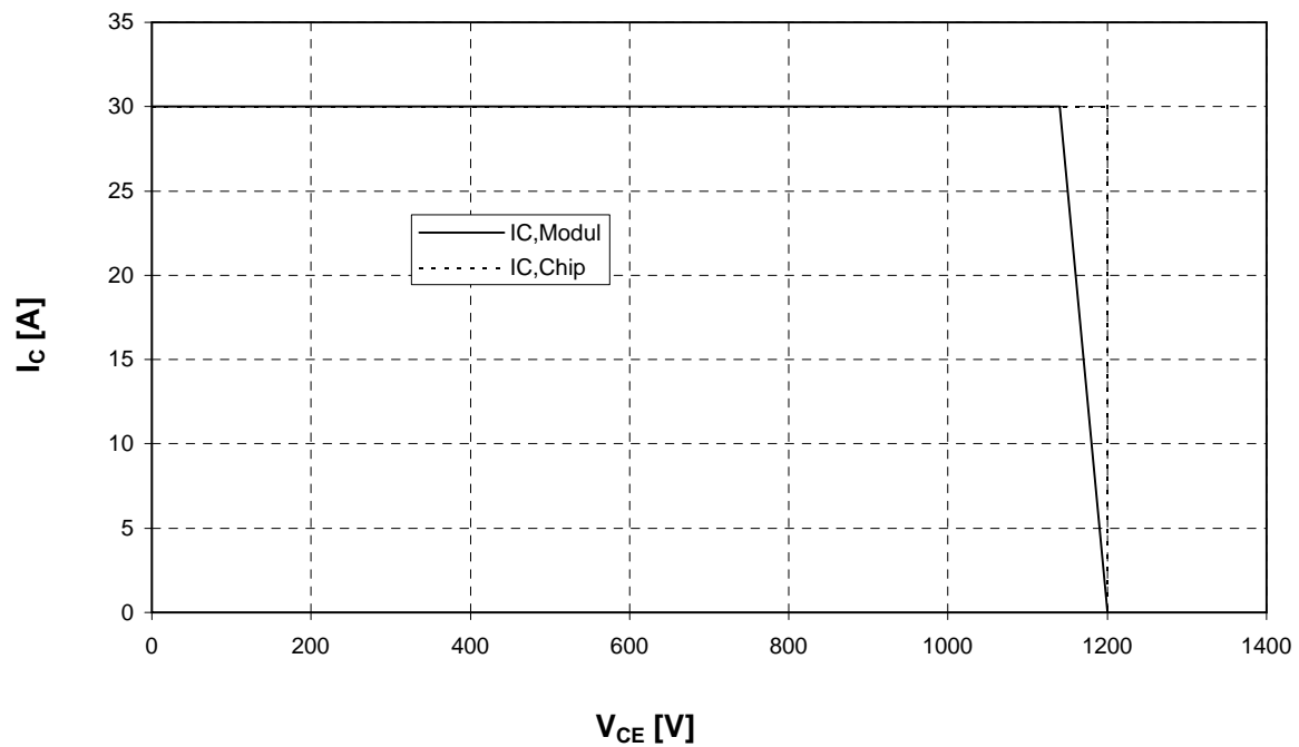
Sicherer Arbeitsbereich Wechselr. (RBSOA) I_c = f(V_{CE}) Reverse bias save operating area Inverter (RBSOA) T_{vj} = 125^\circ\text{C}, V_{GE} = \pm 15\text{V}, R_G = 47 \text{ Ohm}
