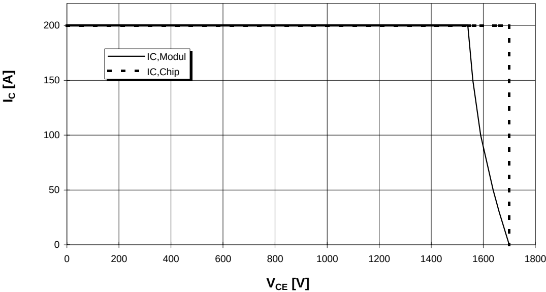
Sicherer Arbeitsbereich (RBSOA) Reverse bias safe operation area (RBSOA)
