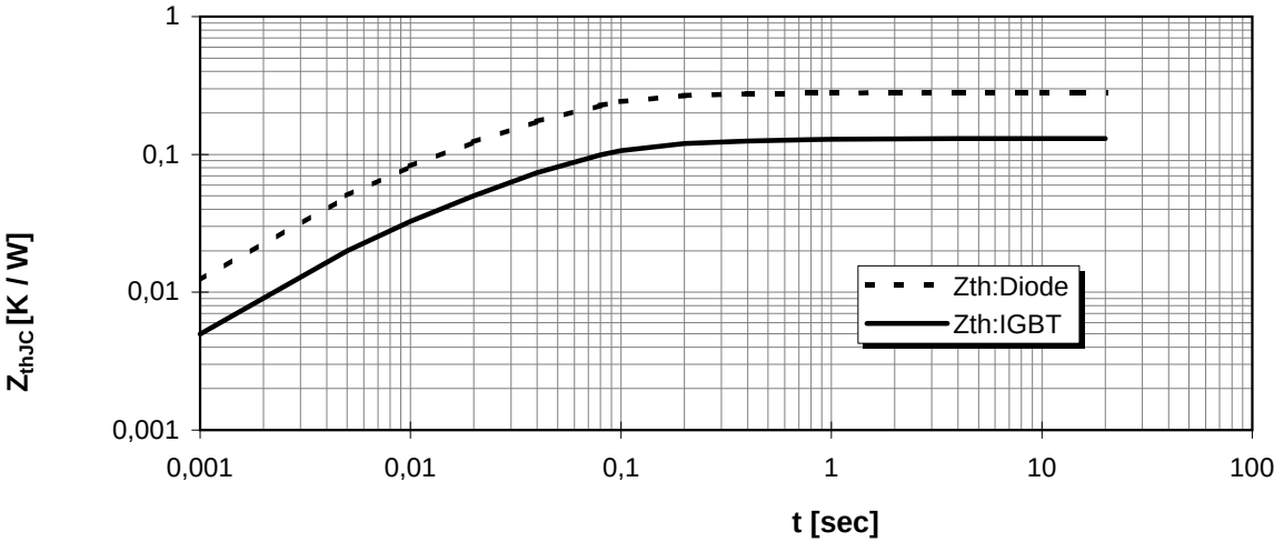
Transienter Wärmewiderstand Transient thermal impedance
