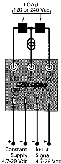
D2415-C, D2440-C DC CONTROL, AC OUTPUT
