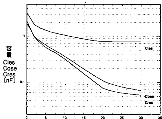
容量-コレクタ・エミッタ間電圧特性 ( T_j=25^\circ\text{C} ) <ブレーキ部> Capacitance vs. Collector-Emitter voltage <BRAKE>
