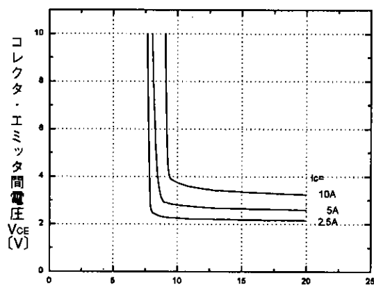
ゲート・エミッタ間電圧 V_{GE} [V] コレクタ・エミッタ間電圧-ゲート・エミッタ間電圧特性 ( T_j=25^\circ\text{C} ) <ブレーキ部> Collector-Emitter voltage vs. Gate-Emitter voltage <BRAKE>
