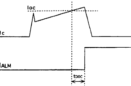
過電流遮断遅れ時間 (tdoc) の定義 Fig.2 Definition of OC delay time
