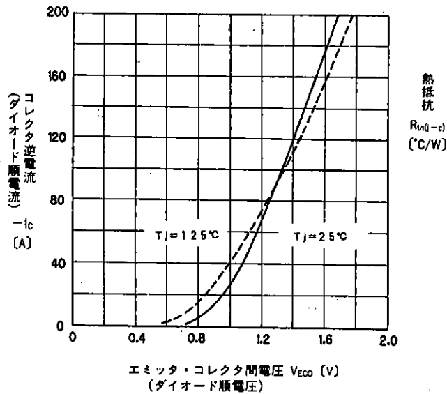
高速フリーホイリングダイオード順電圧 Forward Voltage of Free Wheeling Diode
