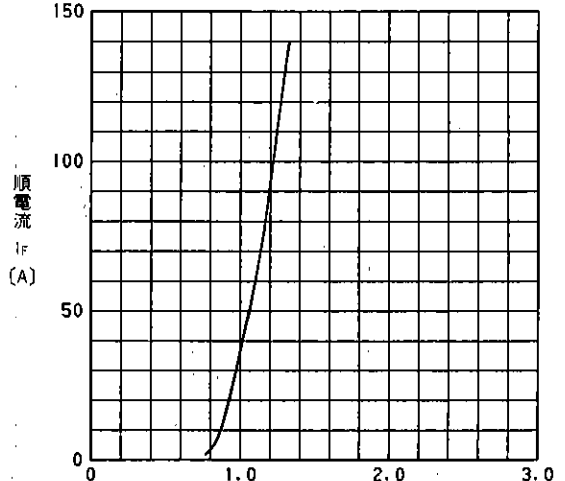
ツェナーダイオード順電圧特性 Forward Voltage Characteristics of Zener Diode
