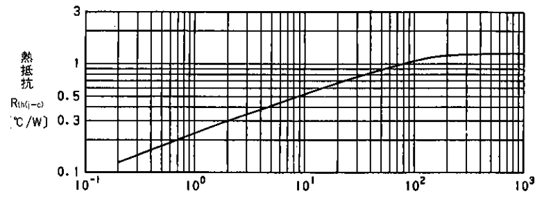
時間 t (msec) 過渡熱抵抗(ツェナーダイオード)特性 Transient Thermal Resistance (Zener Diode)
