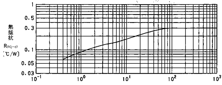
時間 t (sec) 過渡熱抵抗(ダイオード)特性 Transient Thermal Resistance (F.R.D)
