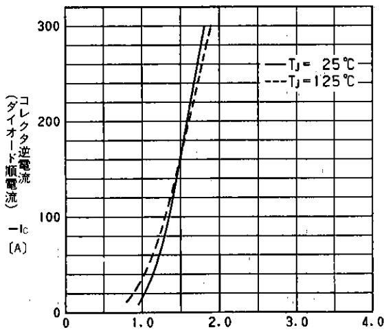
エミッタ・コレクタ間電圧 V_{CEO} (V) (ダイオード順電圧) 高速フリーホイリングダイオード順電圧特性 Forward Voltage of Free Wheeling Diode
