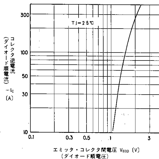
エミッタ・コレクタ間電圧 V_{\text{ECO}} (V) (ダイオード順電圧) 高速フリーホイーリングダイオード順電圧 Forward Voltage of Free Wheeling Diode
