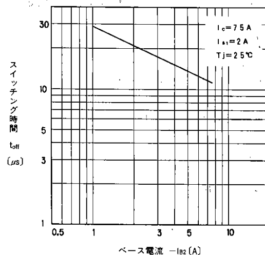
ベース電流 -I_{\text{B2}} (A) スイッチング時間—ベース電流特性 Switching Time
