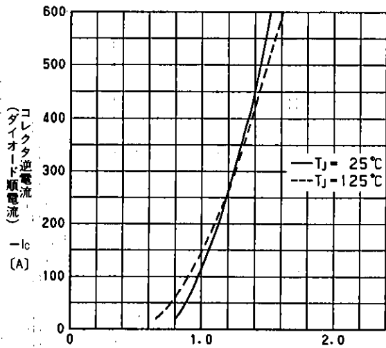
エミッタ・コレクタ間電圧 V_{ceo} (V) (ダイオード順電圧) 高速フリーホイリングダイオード順電圧特性 Forward Voltage of Free Wheeling Diode
