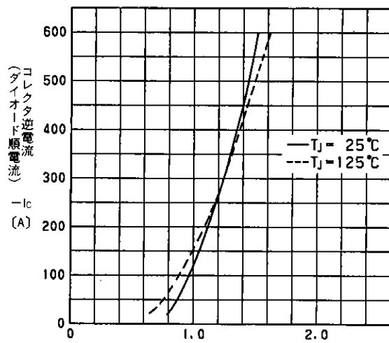
エミッタ・コレクタ間電圧 V_{eco} (V) (ダイオード順電圧) 高速フリーホイリングダイオード順電圧特性 Forward Voltage of Free Wheeling Diode
